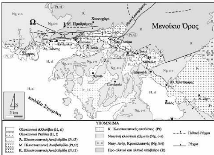
Εικόνα 2. Γεωλογικός χάρτης της ευρύτερης περιοχής Σερρών (τροπ. από Tranos & Mountrakis, 2003)
